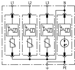
Schemat połączeń DG M TT 320
