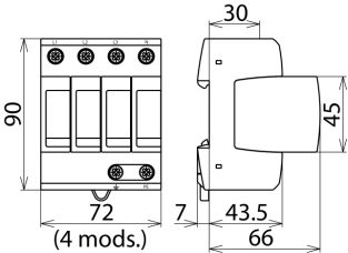
Rysunek wymiarowy DG M TT 320
