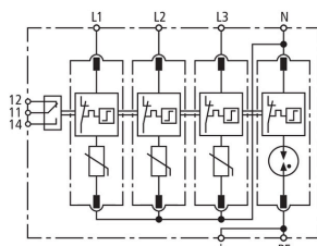
Schemat połączeń DG M TT 385 FM
