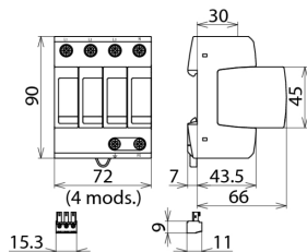
Rysunek wymiarowy DG M TT 385/305 FM
