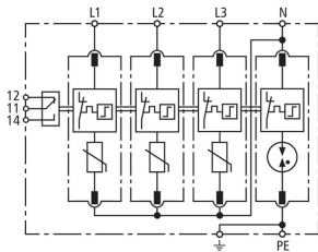
Schemat połączeń DG M TT 385/305 FM
