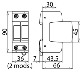
Rysunek wymiarowy DG M TN 150
