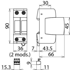
Rysunek wymiarowy DG M TN 275 FM
