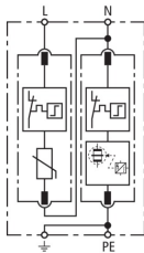
Schemat połączeń DG M H TT 2P 275
