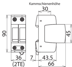
Rysunek wymiarowy DG M H TT 2P 275
