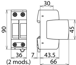
Rysunek wymiarowy DG M TT 2P 385
