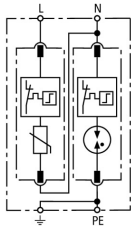
Schemat połączeń DG M TT 2P 385
