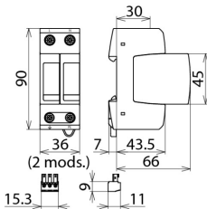
Rysunek wymiarowy DG M TT 2P 275 FM
