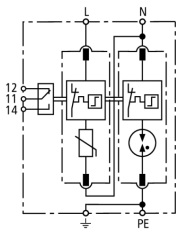
Schemat połączeń DG M TT 2P 275 FM
