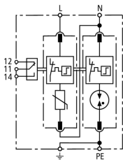
Schemat połączeń DG M TT 2P 320 FM
