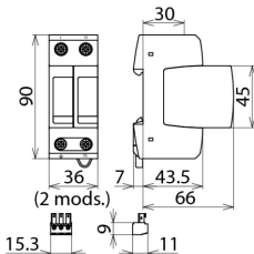
Rysunek wymiarowy DG M TT 2P 320 FM
