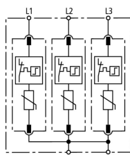
Schemat połączeń DG M WE 600
