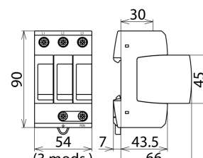
Rysunek wymiarowy DG M WE 600
