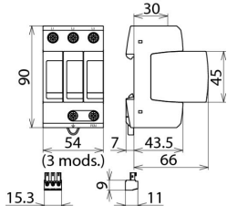
Rysunek wymiarowy DG M WE 600 FM
