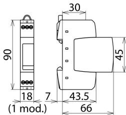
Rysunek wymiarowy DR M 2P 30
