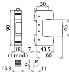
Rysunek wymiarowy DR M 2P 30 FM
