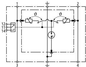
Schemat połączeń DR M 2P 60 FM
