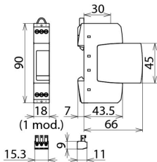
Rysunek wymiarowy DR M 2P 60 FM
