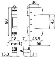
Rysunek wymiarowy DR M 2P 75 FM
