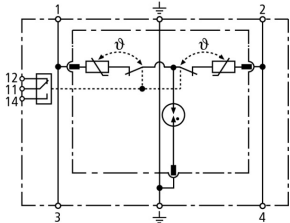
Schemat połączeń DR M 2P 75 FM
