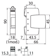
Rysunek wymiarowy DR M 2P 255 SN1803FM
