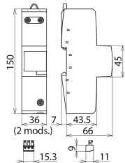
Rysunek wymiarowy DBM 1 760 FM
