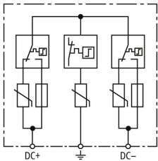
Schemat połączeń DCU YPV SCI 1000 1M
