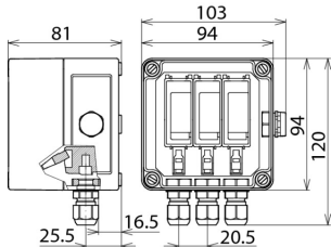
Rysunek wymiarowy DCU YPV SCI 1000 1M
