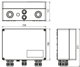
Rysunek wymiarowy DCU 2 YPV 1100 2M 1S
