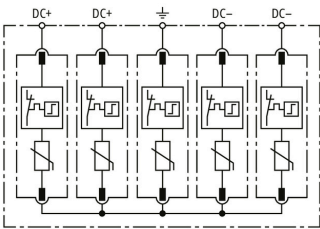
Schemat połączeń DCU 2 YPV 1100 2M 2S
