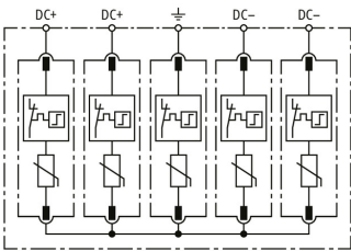
Schemat połączeń DCU 2 YPV 1+2 1000 2M 2S FM
