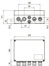
Rysunek wymiarowy DCU 2 YPV 1+2 1000 2M 2S FM
