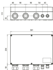
Rysunek wymiarowy DCU 2 YPV 1+2 1000 3M 2S FM
