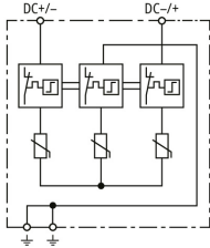
Schemat połączeń DCU 2 YPV 1+2 1000 3M 2S FM
