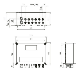
Rysunek wymiarowy DCU 2 YPV 1100 3M 1S MC4 FM
