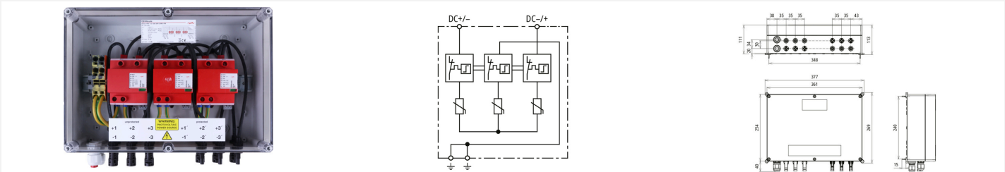
Ilustracja nie są wiążące Schemat połączeń DCU 2 YPV 1+2 1200 3M 1S MC4 Rysunek wymiarowy DCU 2 YPV 1+2 1200 3M 1S MC4 Skrzynka przyłączeniowa generatora do instalacji fotowoltaicznych do 1200 V DC do ochrony trzech wejść MPP i po jednym stringu.
