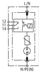
Schemat połączeń DG SE H 1000 VA FM
