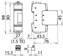
Rysunek wymiarowy DG SE H 1000 VA FM
