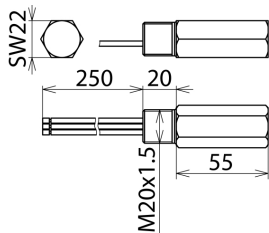
Rysunek wymiarowy DPI CD EXI 24 M
