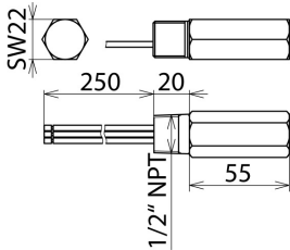
Rysunek wymiarowy DPI CD EXI 24 N
