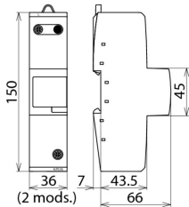
Rysunek wymiarowy DVCI 1 255
