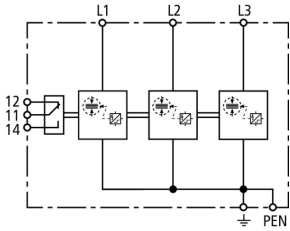
Schemat połączeń DSH TNC 255 FM
