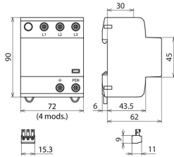
Rysunek wymiarowy DSH TNC 255 FM
