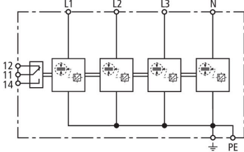
Schemat połączeń DSH B TNS 255 FM
