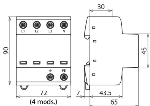
Rysunek wymiarowy DSH TT 255
