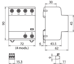
Rysunek wymiarowy DSH B TT 255 FM
