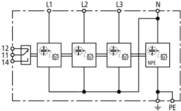
Schemat połączeń DSH B TT 255 FM
