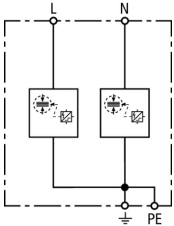
Schemat połączeń DSH TN 255
