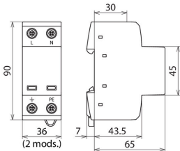
Rysunek wymiarowy DSH TN 255
