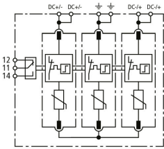
Schemat połączeń DG M YPV 1500 FM
