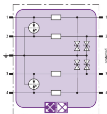
Schemat połączeń BXT ML4 BE 180
