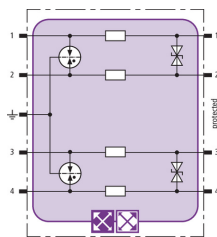
Schemat połączeń BXT ML4 BD 5
