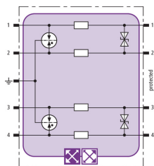
Schemat połączeń BXT ML4 BD 12
