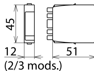
Rysunek wymiarowy BXT ML4 BD 24
