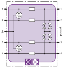
Schemat połączeń BXT ML4 BC 5
