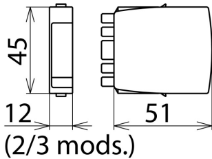
Rysunek wymiarowy BXT ML4 BC 5
