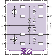
Schemat połączeń BXT ML4 BE C 24
