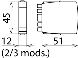
Rysunek wymiarowy BXT ML4 BE C 24
