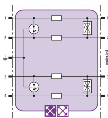
Schemat połączeń BXT ML4 BD HF 24
