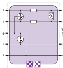
Schemat połączeń BXT ML2 BD HFS
