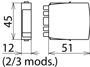
Rysunek wymiarowy BXT ML2 BD S 15
