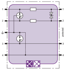
Schemat połączeń BXT ML2 BD S 15
