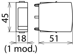
Rysunek wymiarowy DR MOD 60
