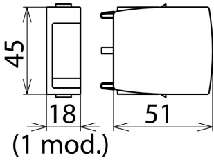
Rysunek wymiarowy DR MOD 75
