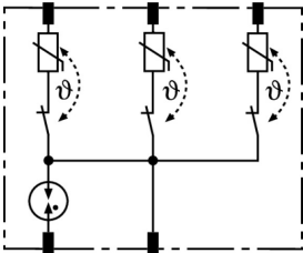
Schemat połączeń DR MOD 4P 255
