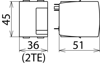
Rysunek wymiarowy DR MOD 4P 255 SN1871
