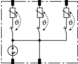
Schemat połączeń DR MOD 4P 255 SN1871
