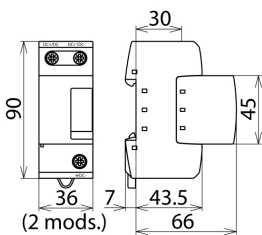
Rysunek wymiarowy DSE M 1 220
