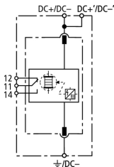
Schemat połączeń DSE M 1 242 FM
