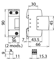
Rysunek wymiarowy DSE M 1 242 FM
