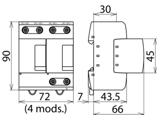
Rysunek wymiarowy DSE M 2P 60
