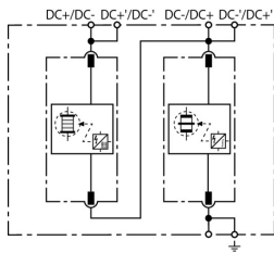
Schemat połączeń DSE M 2P 60
